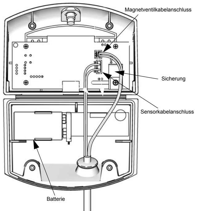
ABB. 11. Einbauort von Batterie und Sicherung im DataTrak-Modul
